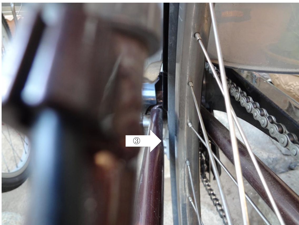
③後ろから車輪をのぞき、矢印の位置の左右の隙間が同じかどうか調べる
